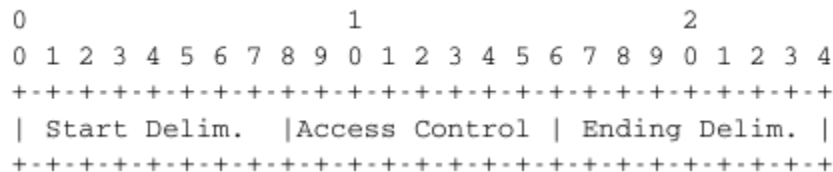
Fig. 75: 802.5 token format
