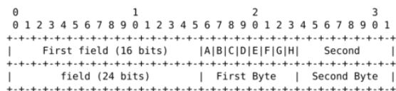
Fig. 38: Message format
