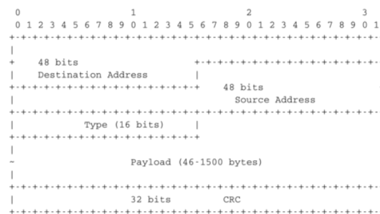
Fig. 82: Ethernet DIX frame format
